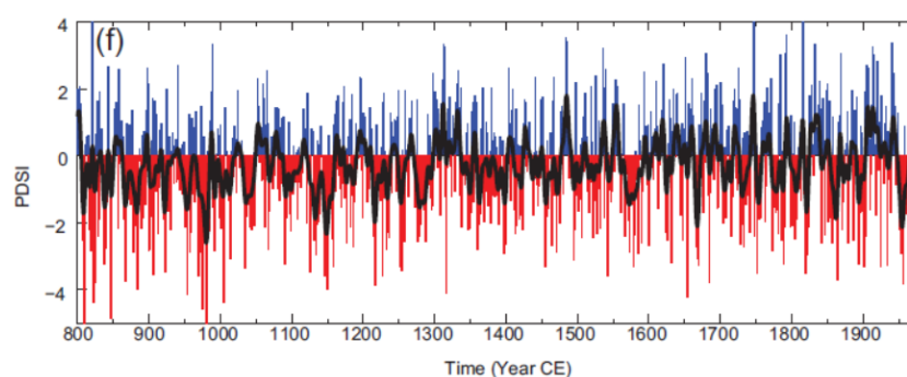
10. ábra: Aszályindex az USA délnyugati részén.
